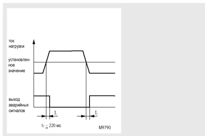
Обнаружение повышенного тока, вариант/002
