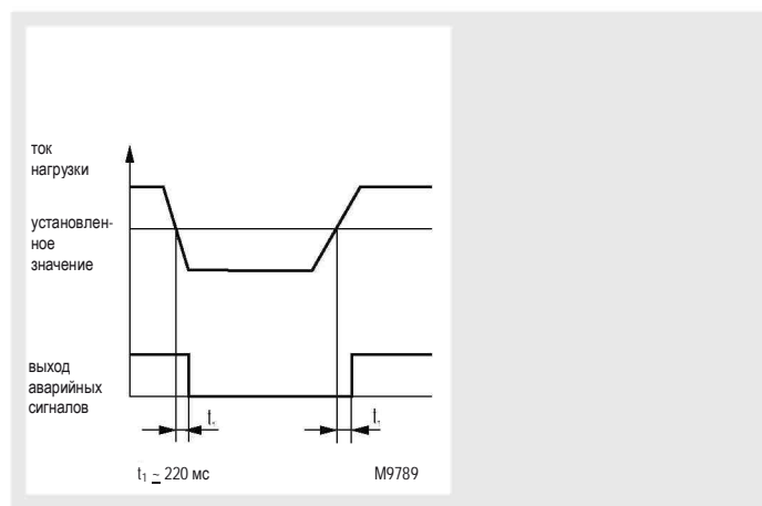
Обнаружение пониженного тока, вариант/001
